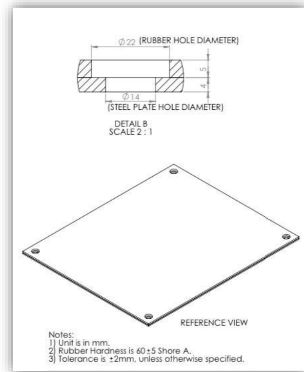
Rajah 3.3: Ukuran bagi saiz lubang pada plat.
