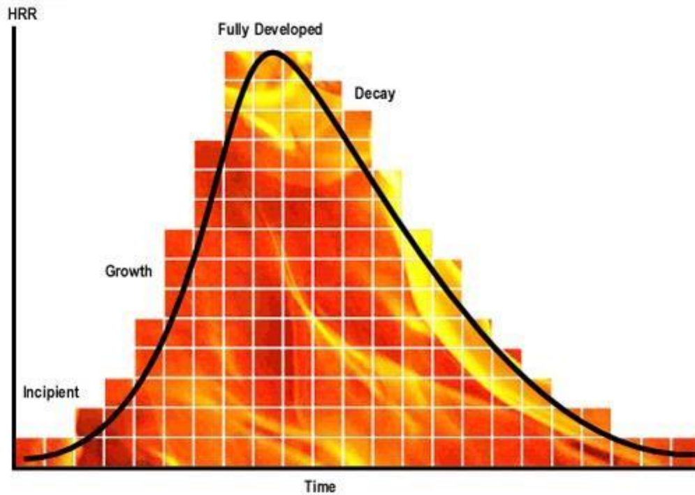
Rajah 2.5.2 Graf Perkembangan Api
